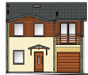
ELEWACJA FRONTOWA
