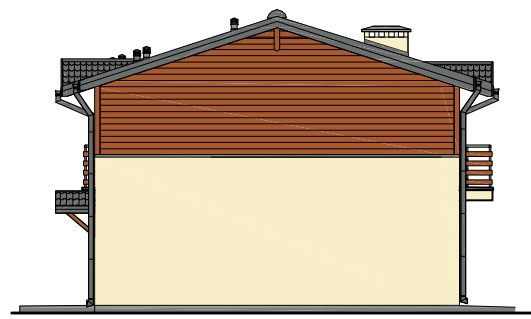
ELEWACJA BOCZNA
