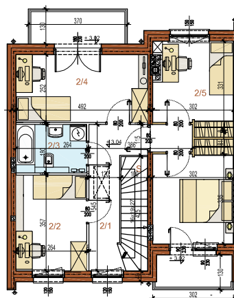
PIĘTRO wariant 3
