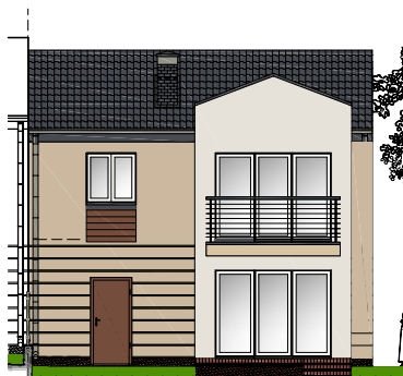
ELEWACJA OGRODOWA
