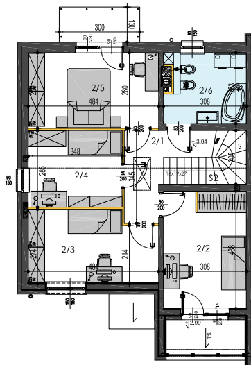
RZUT PIĘTRA WARIANT 3
