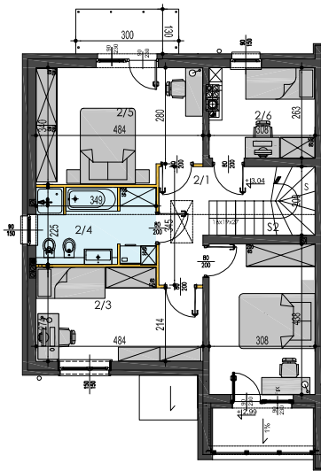
RZUT PIĘTRA WARIANT 2
