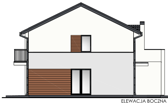
ELEWACJA BOCZNA
